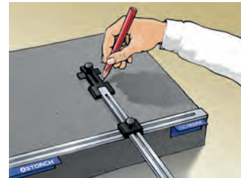
4. Übertragung der Maße auf die Dämmplatte
