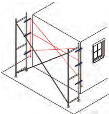
Installation eines ISO DIST Grund-Sets in einem Gerüstsegment
