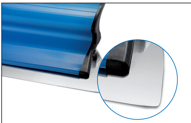
Flexibles Edelstahlblatt mit abgerundeten Ecken für glattes Abziehen mit sehr geringer Nacharbeit.
